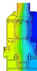
BSF70 Termička provodljivost
