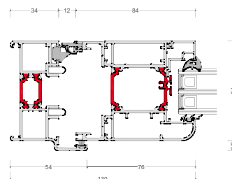
BSF70 Visoka donja vodilica
