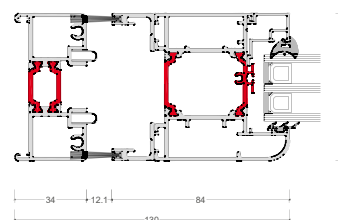
BSF70 Niska donja vodilica
