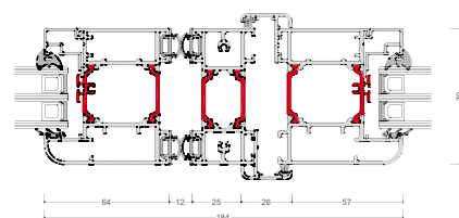
BSF70 Spoj krila i što-ka
