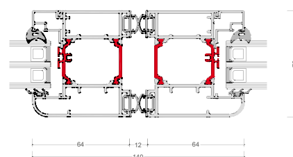
BSF70 Centralni spoj krila
